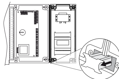
esempio con UltraCella + modulo Ultra EVD
