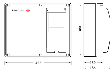
Modulo Ultra 3ph evaporatore e Modulo Ultra 3ph full
